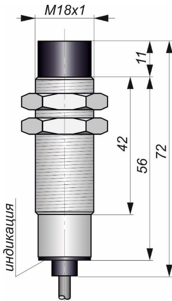
Габаритный чертеж
